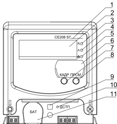
Рисунок 2.2 – Конструкция счетчика.
